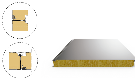
Solape lateral (sistema de fijación vista) Side lap (visible fixation system)
