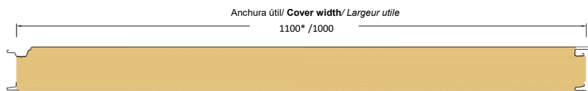
Solape lateral (sistema de fijación vista) Side lap (visible fixation system)
