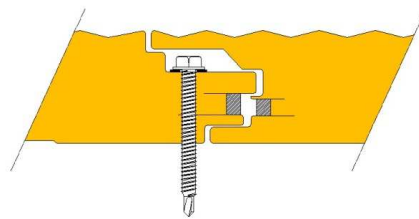
Sección Machihembrado (fija. oculta)
