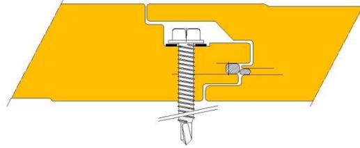
Recouvrement longitudinal (fixations secrètes)
