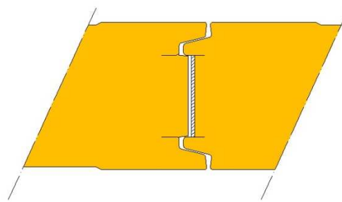
Sección Machihembrado (fija. oculta)
