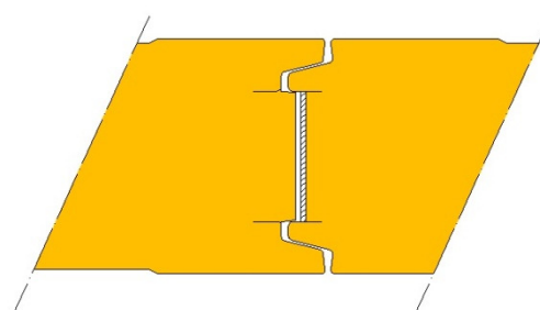
Sección Machihembrado (fija. oculta)
